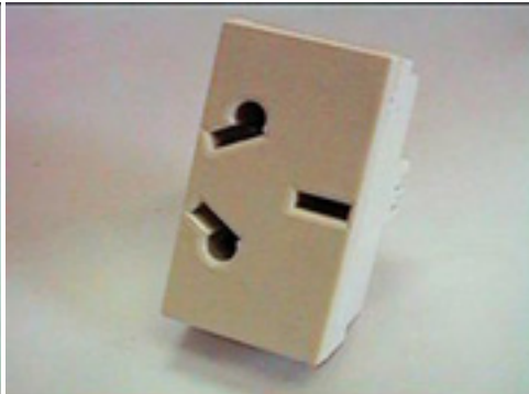
Módulo de tomacorriente bi-norma de la línea HABITAT 10 A - 250 V.
